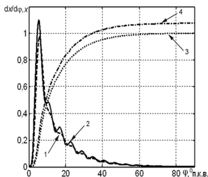
Рисунок 6 – Зависимость изменения моделируемых нормированных характеристик тепловыделения x (3, 4) и скорости тепловыделения dx/d\varphi (1, 2) в цилиндре дизеля 4Ч 11/12,5 от угла поворота коленчатого вала \varphi : 1, 3 – без присадки в топливе; 2, 4 – с присадкой в топливе декаква-2-сульфобензоат эрбия
