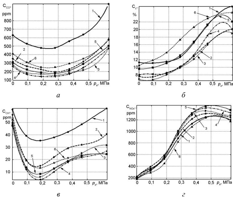
Рисунок 3 – Экспериментальные зависимости изменения концентраций: a – оксида углерода C_{CO} ; б – сажи C_c ; в – углеводородов C_{CH} ; г – оксидов азота C_{NOx} в отработавших газах дизеля 4Ч 11/12,5, работающего на топливе с присадкой декаква-2-сульфобензоат эрбия, от изменения среднего эффективного давления p_e дизеля при заданных значениях частоты вращения: 1 – n = 1000 \text{ мин}^{-1} ; 2 – n = 1400 \text{ мин}^{-1} ; 3 – n = 1600 \text{ мин}^{-1} ; 4 – n = 1800 \text{ мин}^{-1} ; 5 – n = 2000 \text{ мин}^{-1} ; 6 – n = 2200 \text{ мин}^{-1}
