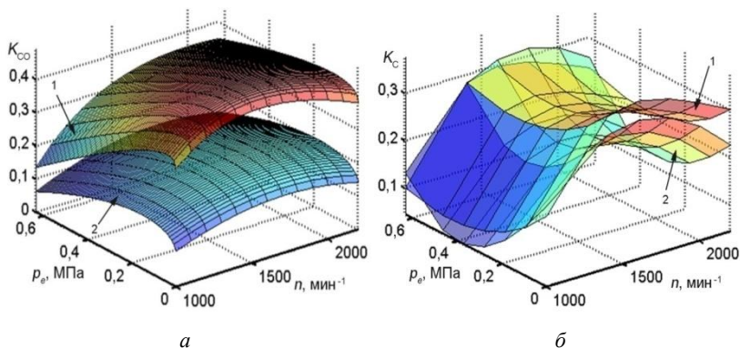
Рисунок 11 – Расчётные зависимости коэффициентов выхода: а – оксида углерода CO; б – сажи С с отработавшими газами от изменения частоты вращения n и среднего эффективного давления p_e дизеля 4Ч 11/12,5 при работе на топливе с присадками: 1 – декаква-2-сульфобензоат эрбия; 2 – гидроксокарбонат лантана
