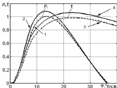
Рисунок 7 – Зависимости изменения нормированного давления рабочего тела p_i и нормированной индикаторной температуры T_i от угла поворота коленчатого вала в первом цилиндре дизеля 4Ч 11/12,5 (экспериментальные индикаторные диаграммы): 1, 3 – топливо без присадки; 2, 4 – топливо с присадкой декааква-2-сульфобензоат эрбия
