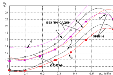
Рисунок 10 – Экспериментальные зависимости концентрации сажи в ОГ дизеля 4Ч 11/12,5, работающего на топливе без присадки, с присадками гидроксокарбонат лантана и декаква-2-сульфобензоат эрбия, от изменения среднего эффективного давления P_e при заданных значениях частоты вращения: 1, 2, 3 – n = 1600 \text{ мин}^{-1} ; 4, 5, 6 – n = 2000 \text{ мин}^{-1}
