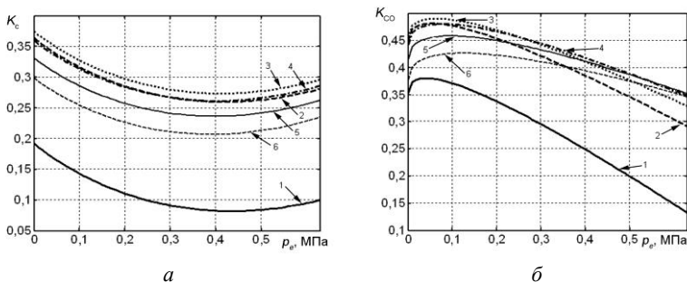
Рисунок 4 – Расчётные зависимости коэффициентов выхода: а – сажи K_c , б – оксида углерода K_{CO} с отработавшими газами дизеля 4Ч 11/12,5, работающего на топливе с присадкой декаква-2-сульфобензоат эрбия, от среднего эффективного давления p_e при заданных значениях частоты вращения: 1 – n = 1000 мин -1 ; 2 – n = 1400 мин -1 ; 3 – n = 1600 мин -1 ; 4 – n = 1800 мин -1 ; 5 – n = 2000 мин -1 ; 6 – n = 2200 мин -1
