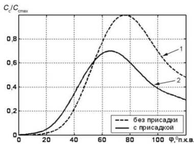
Рисунок 8 – Зависимость изменения моделируемых относительных значений концентрации сажи в цилиндре дизеля 4Ч 11/12,5 от угла поворота коленчатого вала при его работе на номинальном режиме: 1 – без присадки; 2 – с присадкой декааква-2-сульфобензоат эрбия
