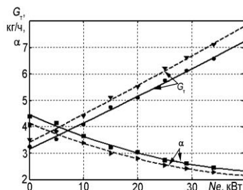
Рисунок 2 – Зависимости изменения часового расхода топлива G_r , коэффициента избытка воздуха \alpha от эффективной мощности Ne дизеля 4Ч 11/12,5 при работе с частотой вращения n = 1800 \text{ мин}^{-1} : ●, ▼, ▲, ■ – данные эксперимента; —, ---- – данные теплового расчёта соответственно с присадкой и без присадки
