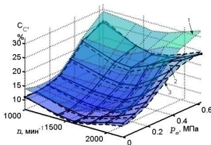
Рисунок 9 – Экспериментальные зависимости концентрации сажи в ОГ от изменения частоты вращения n и среднего эффективного давления P_e дизеля 4Ч 11/12,5 при работе на топливе: 1 – без присадки; 2 – с присадкой гидроксокарбонат лантана; 3 – с присадкой декаква-2-сульфобензоат эрбия
