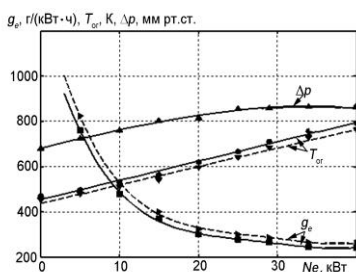
Рисунок 1 – Зависимости изменения удельного эффективного расхода g_e , температуры отработавших газов T_{ог} , перепада давления \Delta p от эффективной мощности Ne дизеля 4Ч 11/12,5 при работе с частотой вращения n = 1800 \text{ мин}^{-1} : ●, ▼, ▲, ■ – данные эксперимента; —, ---- – данные теплового расчёта соответственно с присадкой и без присадки
